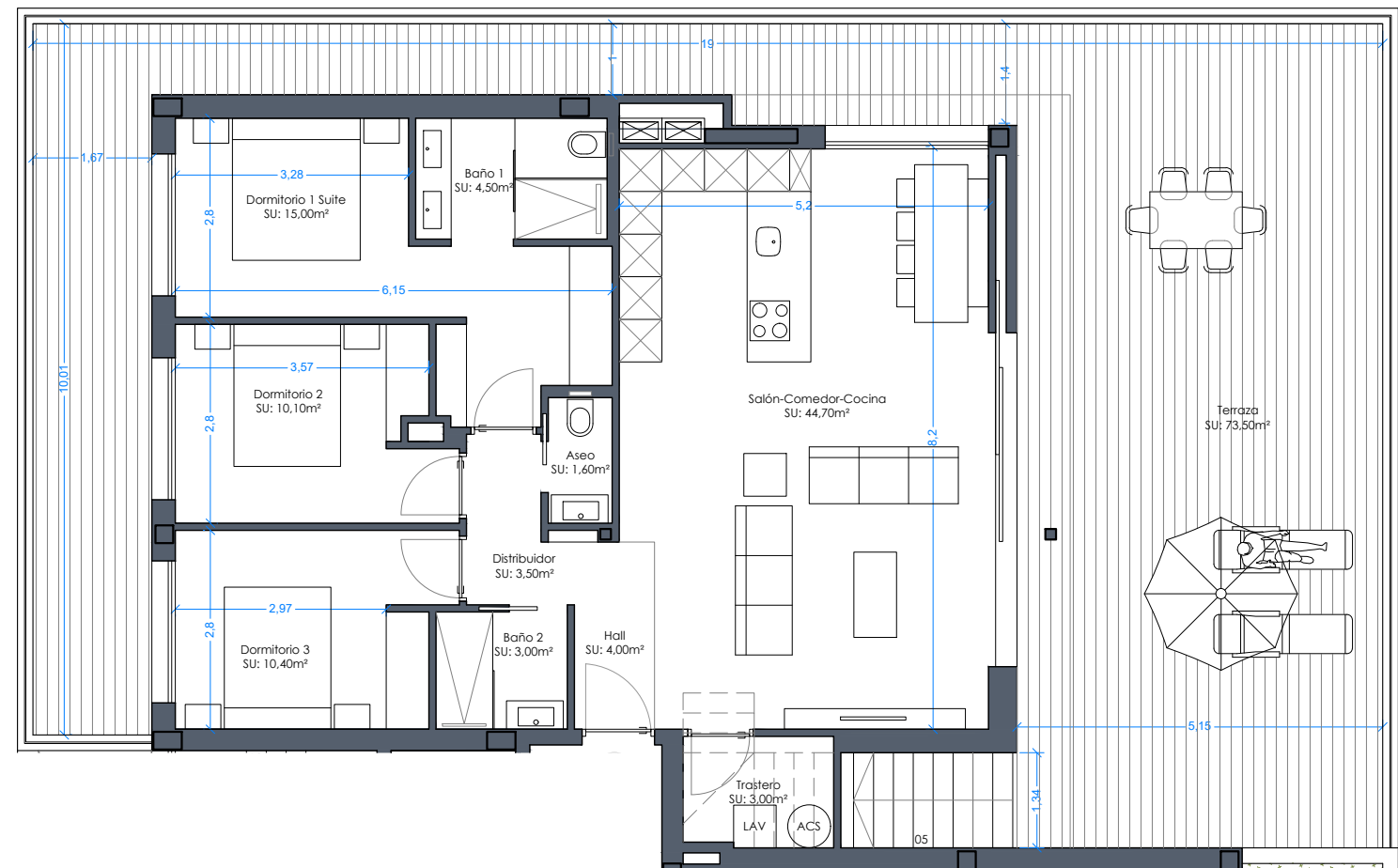
VIVIENDA 17 - ÁTICO
